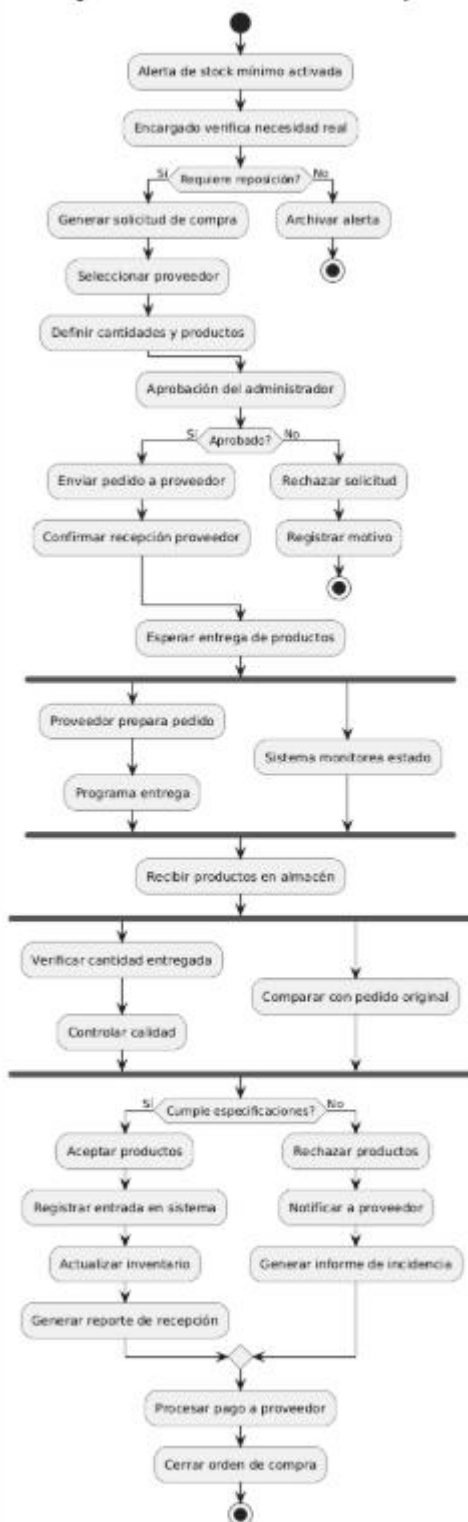
Diagrama de Actividades - Proceso de Compra
